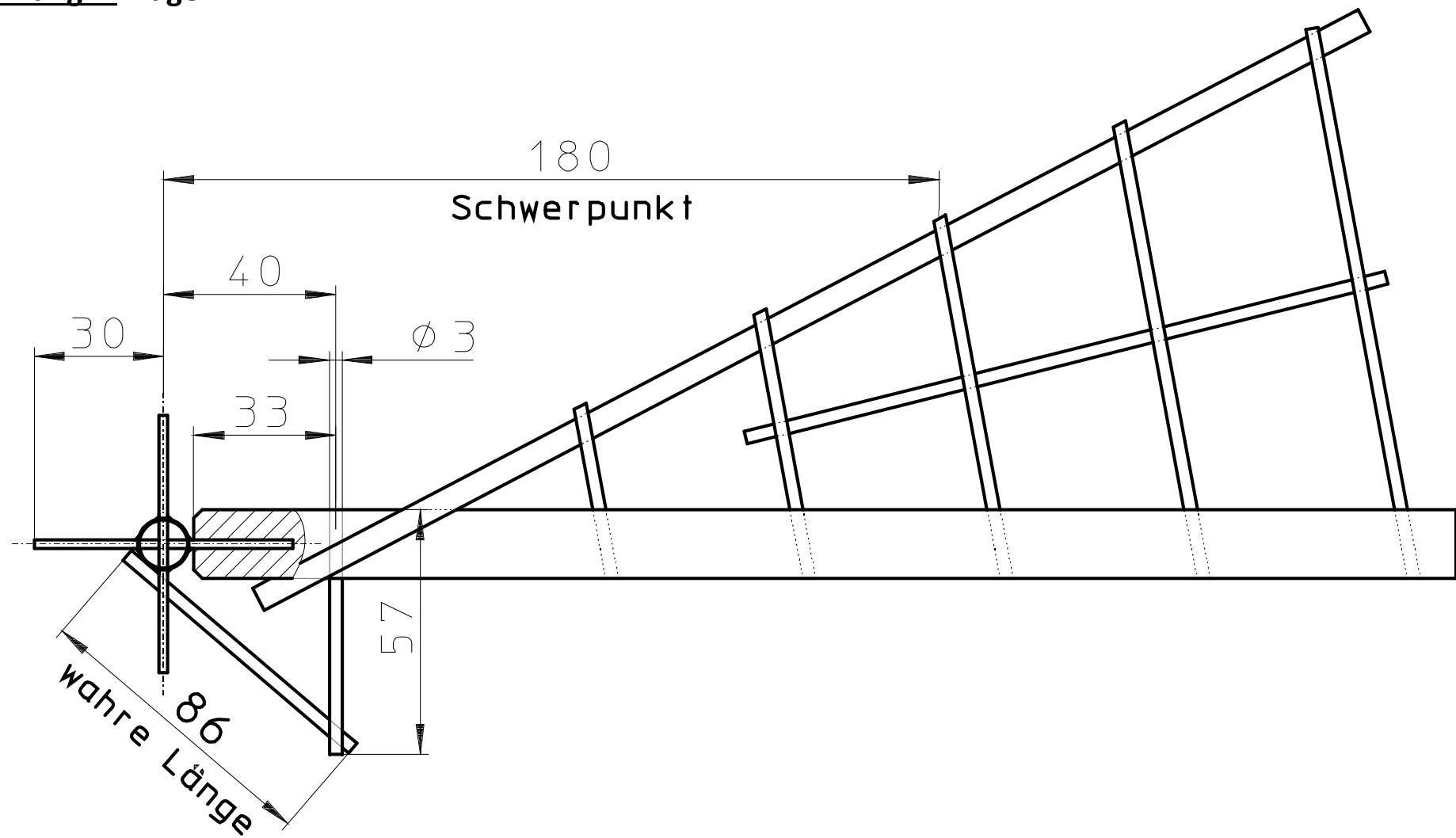
Zeichnung 4: Flügel
